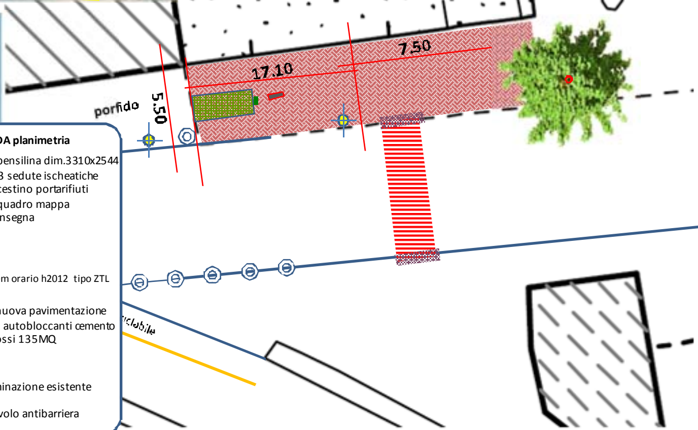
Schema planimetrico
